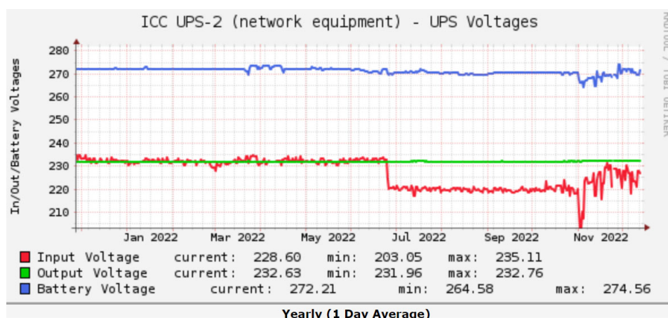
Рис. 10.2. Річний графік вхідної напруги на пристроях безперебійного живлення ІОЦ
